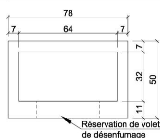
3 parois de 7cm + 1 de 11cm
