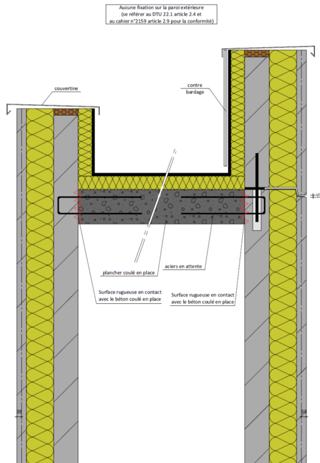
Figure 20 : Panneau porteur – Détail sur acrotère
