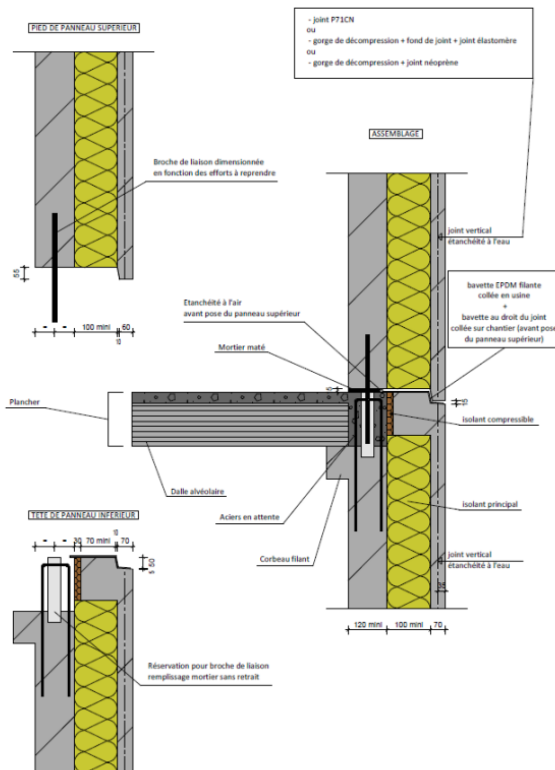
Figure 7 : Panneau porteur – liaison avec plancher avec dalle alvéolaire sur appui corbeau filant - rejingot formé par le béton et l'isolant
