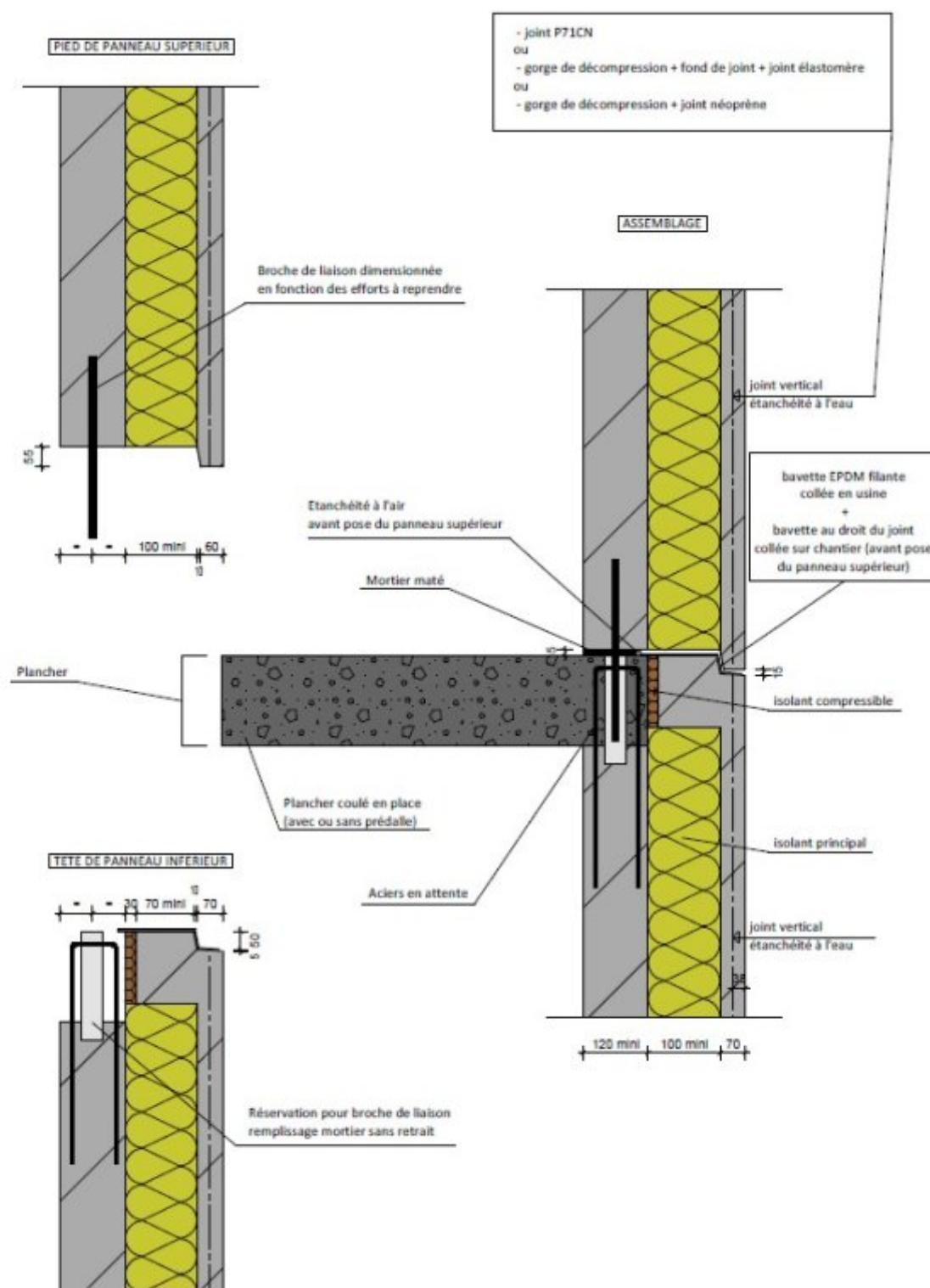
Figure 6 : Panneau porteur – liaison avec plancher coulé en place ou prédalle avec appui (en zone sismique) - rejingot formé par le béton et l'isolant
