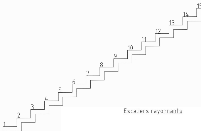
Volées droites à sous-face crémaillère
